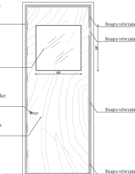
ALZADO FRONTAL
