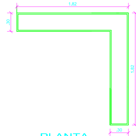
PLANTA MUEBLE EN ACERO INOXIDABLE ESCALA 1:10
