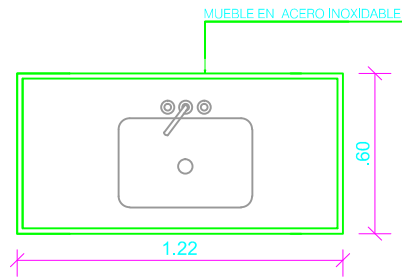
PLANTA MUEBLE EN ACERO INOXIDABLE ESCALA 1:10
