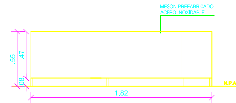
ALZADO MUEBLE EN ACERO INOXIDABLE ESCALA 1:10
