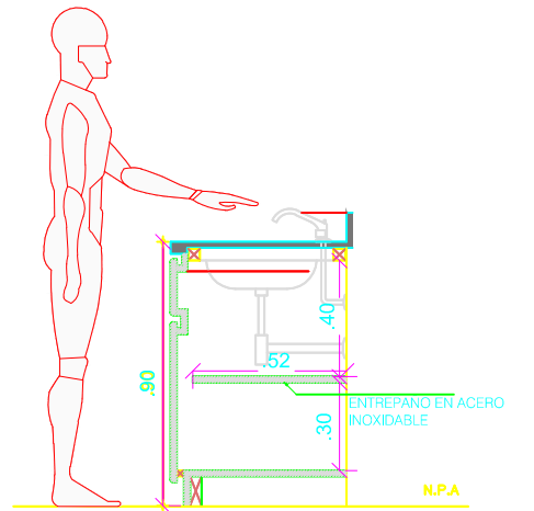
SECCION A-A MUEBLE ACERO INOXIDABLE ESCALA 1:10
