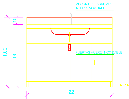
ALZADO MUEBLE EN ACERO INOXIDABLE ESCALA 1:10
