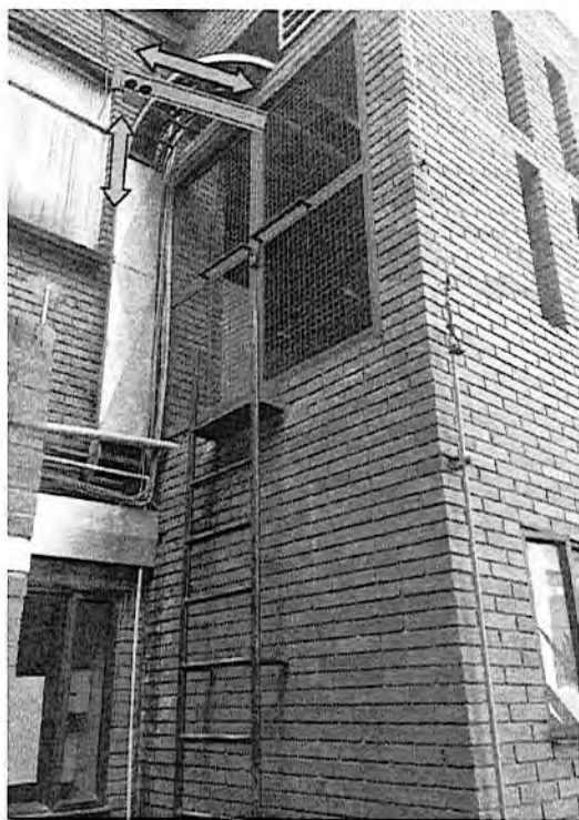
Ubicación del sistema de izaje de cargas con sus sistemas de movimientos de carga.
