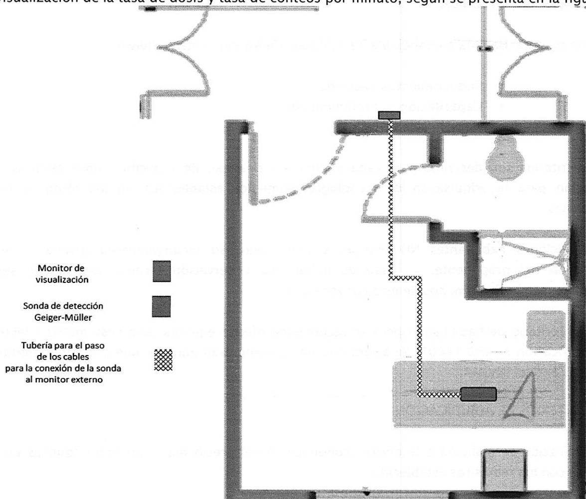
Figura 1. Vista superior de la habitación con el montaje del detector Geiger-Müller en el techo
